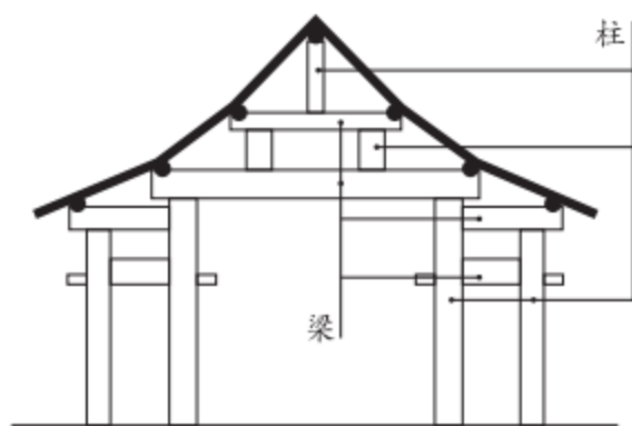
中国古建筑大木构架剖面示意图
